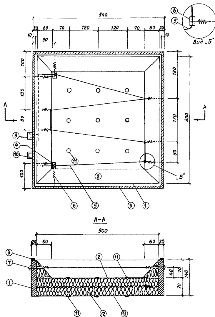
Рисунок А.2. Конструкция прибора площадью 0,25 м 2
