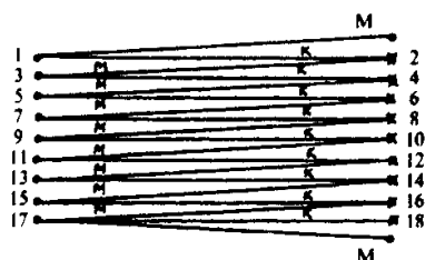
Батарея дифференциальных термопар
